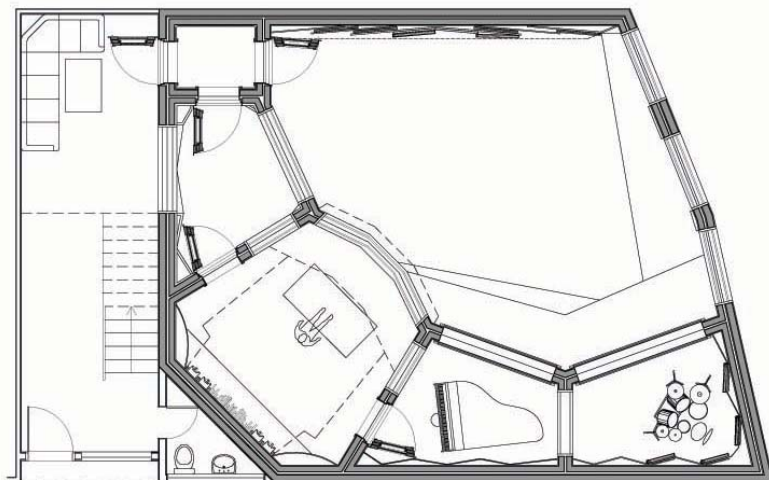
PLANTA DO ESTÚDIO
