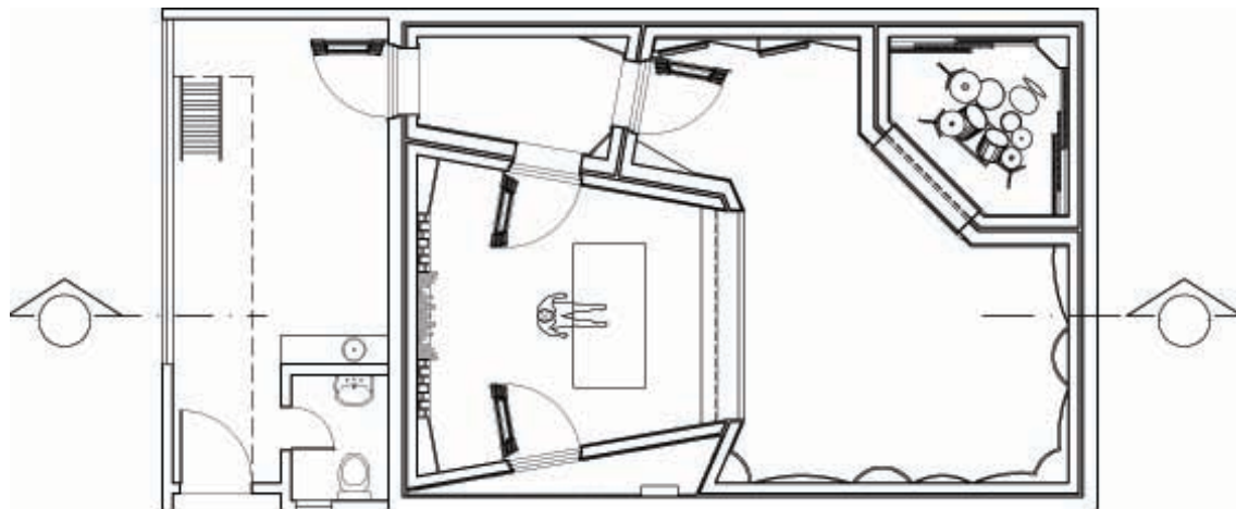
PLANTA DO ESTÚDIO
