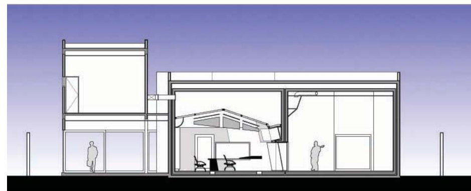
CORTE DO ESTÚDIO
