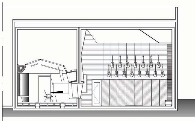
CORTE DO ESTÚDIO
